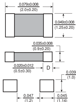
MCB10
