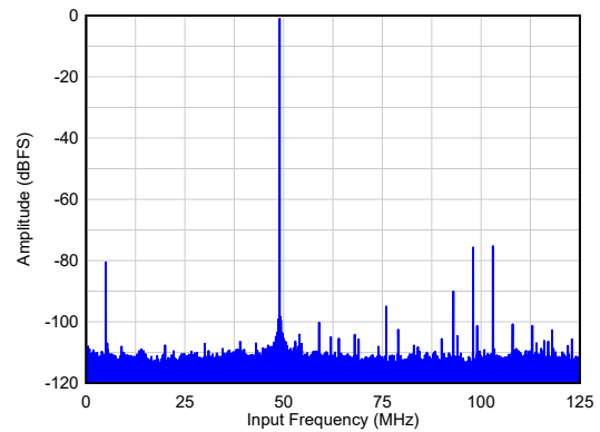
SNR = 70.1dBFS, HD23 = 76dBc, Non HD23 = 80dBFS
