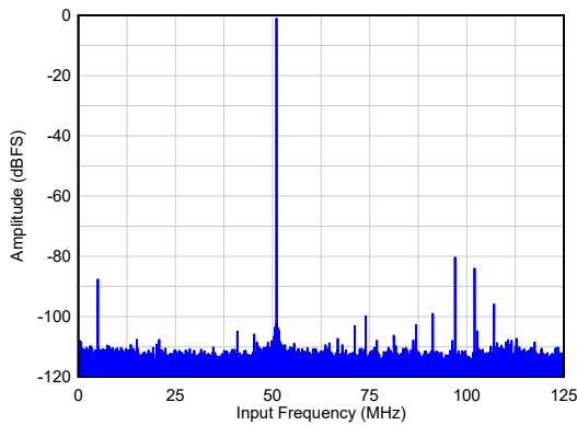
SNR = 71.4dBFS, HD23 = 80dBc, Non HD23 = 85dBFS
