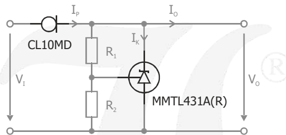
Fig. 3 Spannungsversorgung mit geringem Bauteilbedarf für \mu Controller und andere Schaltungen mit niedrigem Eingangstrom
