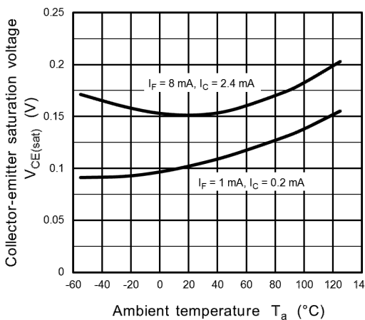
Fig. 11.10 V_{CE(\text{sat})} - T_a
