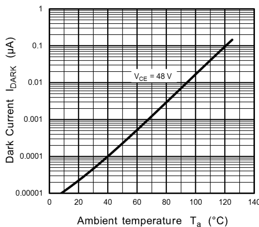
Fig. 11.9 I_{\text{DARK}} - T_a
