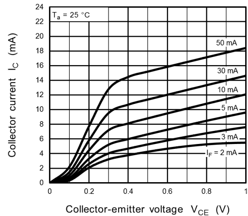
Fig. 11.8 I_C - V_{CE}
