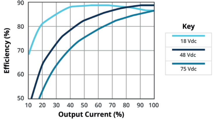
EFFICIENCY VS OUTPUT LOAD PDQ15-Q48-S3-D
