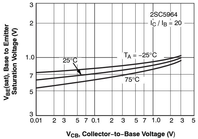
Figure 17. V_{BE(sat)} - I_C
