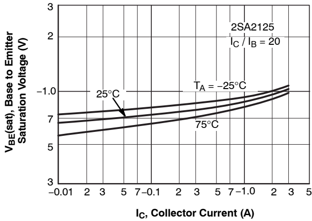
Figure 16. V_{BE(sat)} - I_C
